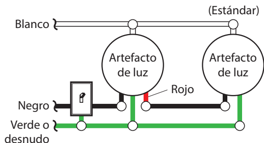
Esquema eléctrico 1
