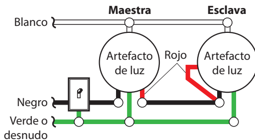
Esquema eléctrico 2
