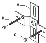
A - (1x) Support de montage B - (2x) Vis de montage du luminaire C - (2x) Ecrou décoratif (Cet élément est fixé à l'endos du couvercle de la lanterne.)
