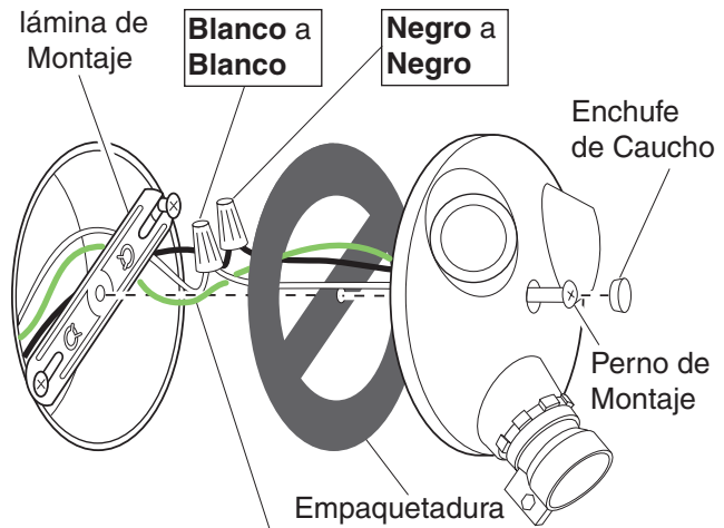
Montaje en alero
