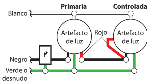
Esquema eléctrico 2
