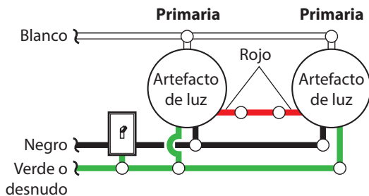
Esquema eléctrico 3
