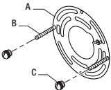
A - (1x) Soporte de montaje B - (2x) Tornillos de montaje del aparato C - (2x) Tuercas decorativas (Este conjunto está sujeto a la parte trasera del farol)
